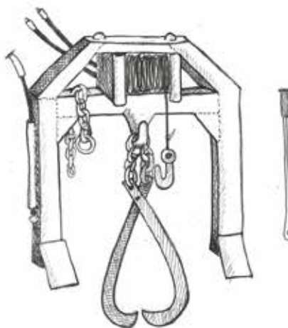
Udrustning til landbrugstraktor: Kævløbue med saks og kæder, spil og kædefisker. De påsatte stykker nederst på kævløbuen kaldes stablesko.
